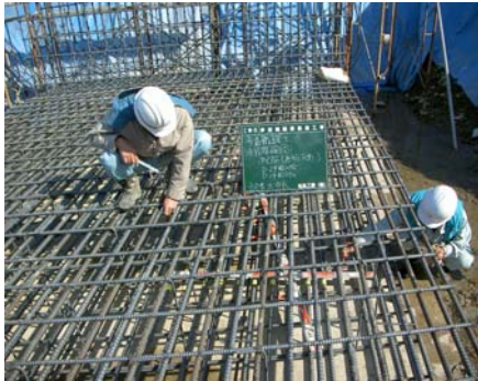
函渠底版鉄筋工確認
